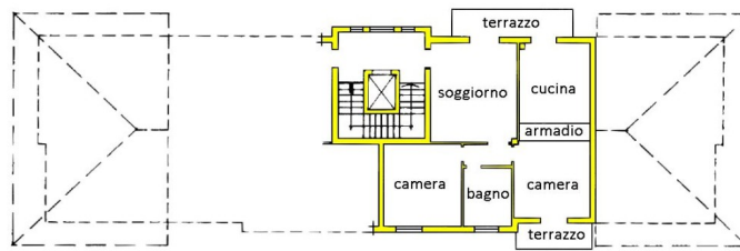
secondo piano
