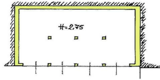
PIANTA PIANO SEMINTERRATO
