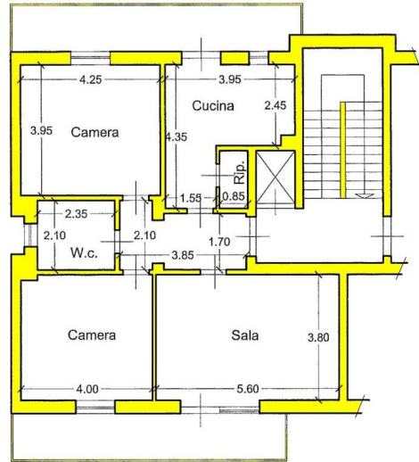
PIANO TERZO
