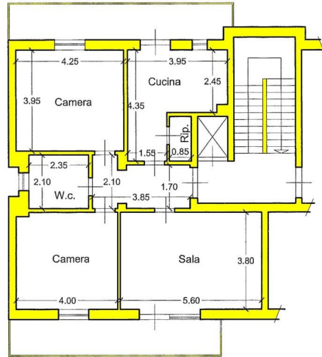
PIANO TERZO
